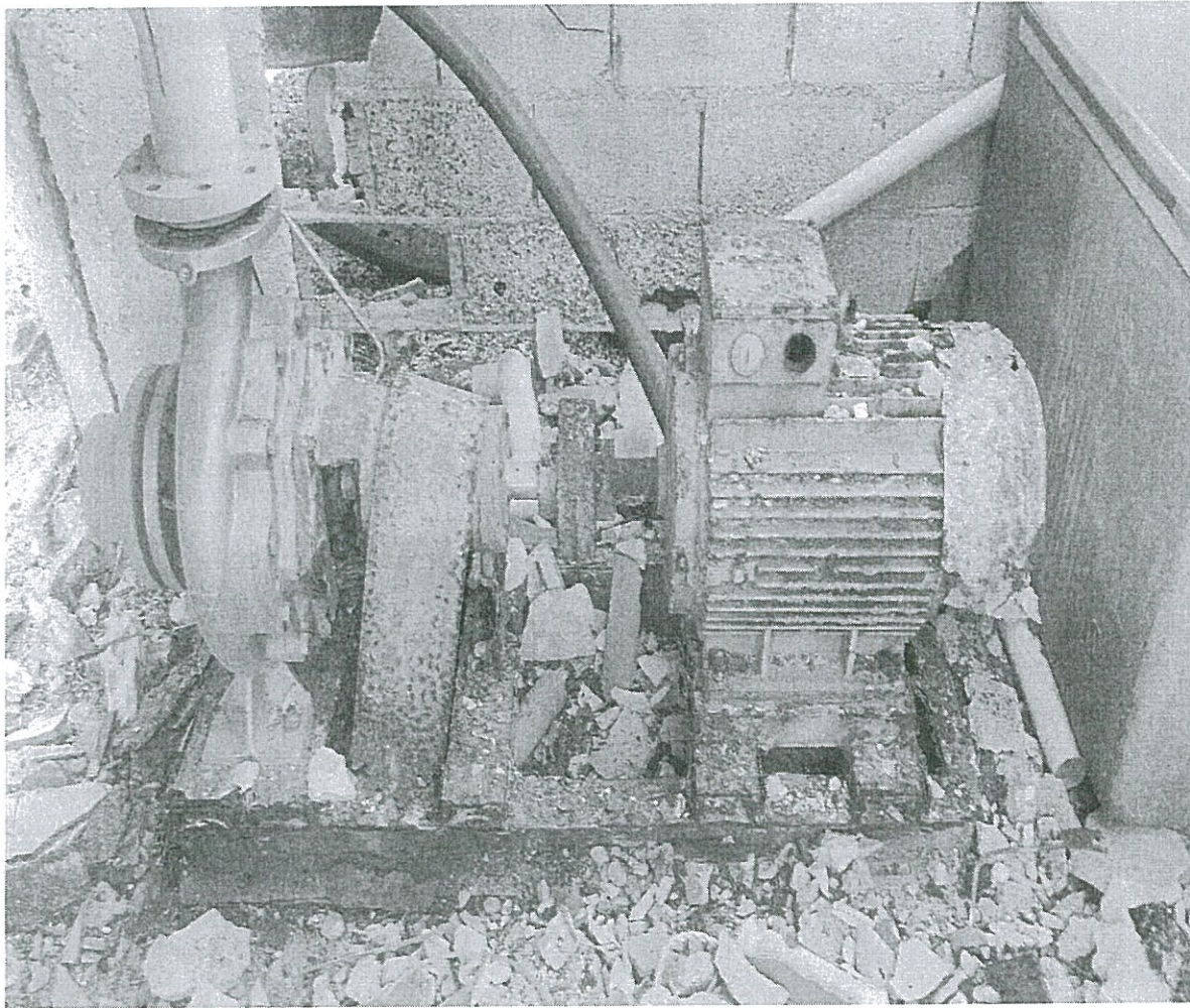
เครื่องสูบน้ำทะเล ขนาดท่อ 4 นิ้ว มอเตอร์ 30 แรงม้า
