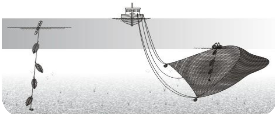
ภาพที่ ๔๒ ลักษณะของเครื่องมืออวนซ้อนปลาจะละเม็ดขณะทำการประมง
