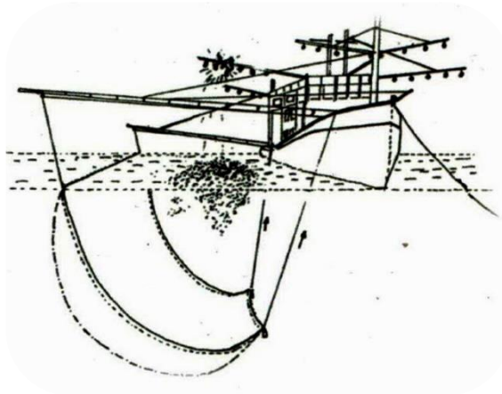
ภาพที่ ๔๕ ลักษณะของเครื่องมืออวนช้อน/ยกปลากระตักขณะทำการประมง (กรมประมง, ๒๕๕๙)
