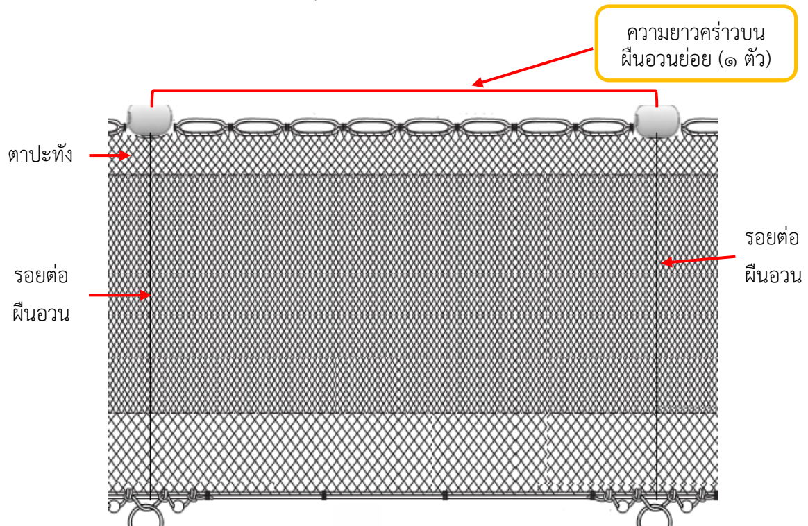
ภาพที่ ๒ ลักษณะฝืนอวนย่อยของอวนล้อมจับและตำแหน่งการวัดความยาว
