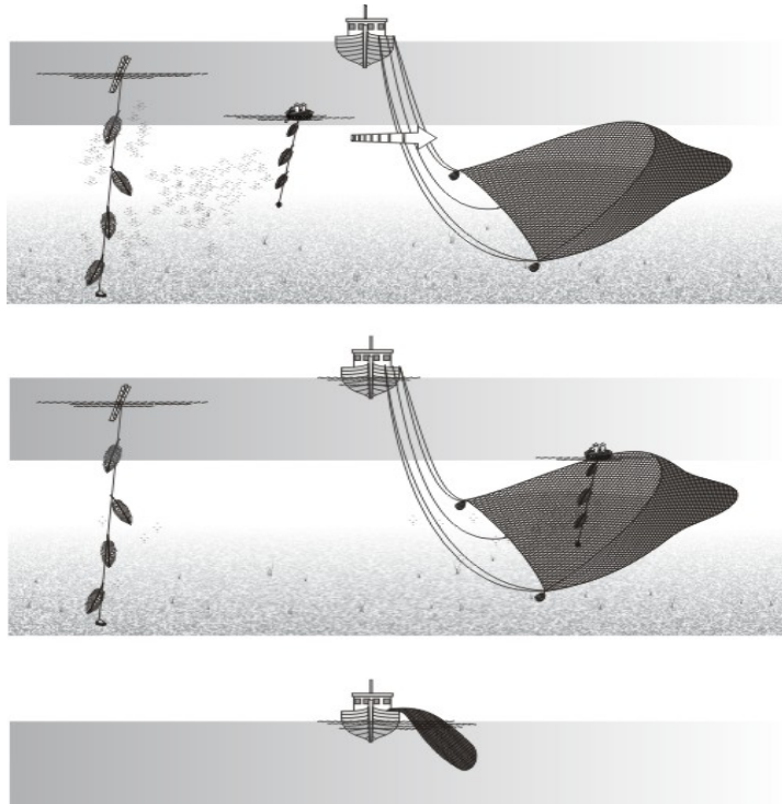
ภาพที่ ๕๔ ลักษณะการทำงานการประมงอวนซ้อนปลาจะละเม็ด
